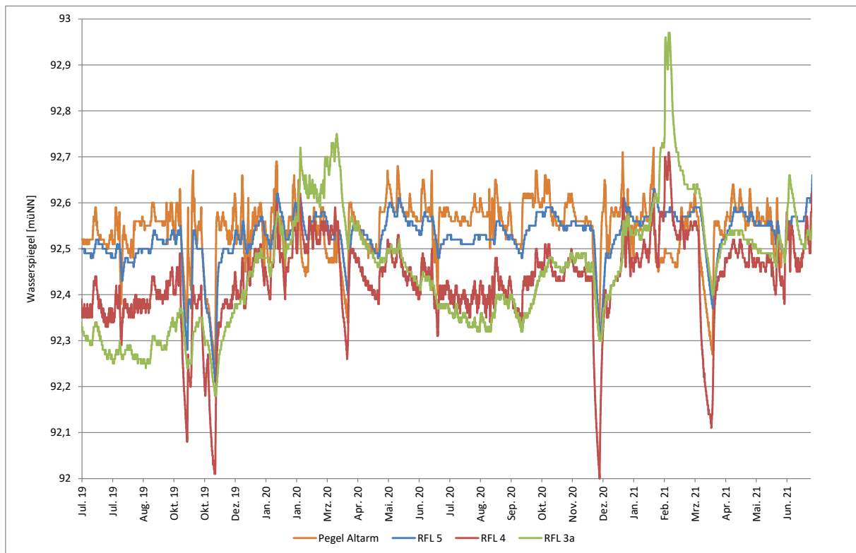
Abb. 3 Grundwasserstandsentwicklung in der Nähe der Siedlung Neufeld seit Sommer 2019
